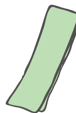
帯揚げ
